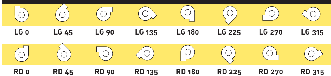
Positions de montage - Vues côté aspiration
